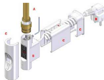
Topná tyč se skládá ze 3 komponentů, je NUTNÉ OBJEDNAT část A + B + C.
