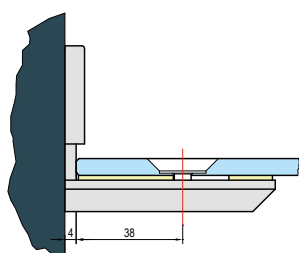
L-kování
