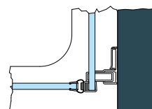
Detail A půdorys:
