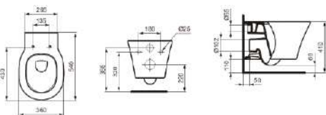
Aquablade - hluboké splachování, 36 x 54 cm, bílé (kód E079601(E005401)) Rimless - hluboké splachování, 36 x 54 cm, bílé (kód E015501.2 (E228801))
