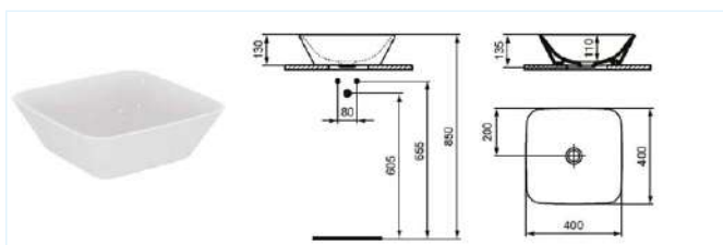
Šířka Hloubka Výška Barva Obj. kód 400 mm 400 mm 130 mm bílá E078601(E034701) 600 mm 400 mm 130 mm bílá E078701(E034801)
