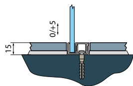
U) Varianta montáže skrytého kotvení pod obklad
