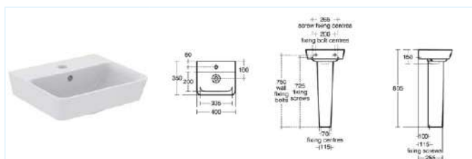
Šířka Hloubka Výška Barva Obj. kód 400 mm 350 mm 150 mm bílá E076901 500 mm 450 mm 160 mm bílá E076801 550 mm 460 mm 160 mm bílá E076701 600 mm 460 mm 160 mm bílá E076601 650 mm 460 mm 160 mm bílá E074101
