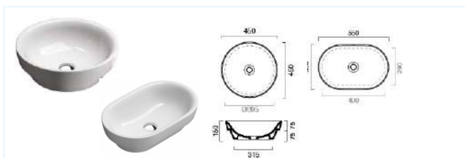
Umyvadlo nábytkové na desku s úpravou Cataglaze
