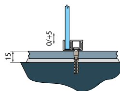
A) Varianta montáže skrytého kotvení na obklad
