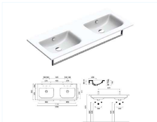
Umyvadlo dvojité nábytkové bez otvoru pro baterii, hranaté s úpravou Cataglaze
