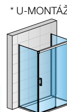
* U-MONTÁŽ CO3ST + CO3S2D + CO3ST Od šířky 1200 mm doporučujeme použít rohové vzpěry 2x RCO.50.1000
