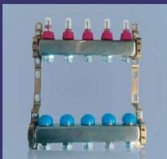
Podlahové vytápění
