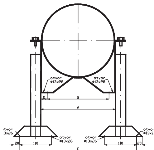
Rozměry pro založení komínu na svislou konstrukci pomocí patní konzoly Typ 325 a Typ 475
