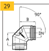
Koleno 90° s KO záplata (se sponou)
