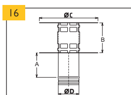
Protidešťová hlavice (bez spony)
