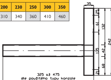
Rozměry pro založení komínu na svislou konstrukci pomocí patní konzoly Typ 325 a Typ 475
