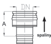
Přechod PPL-PM
