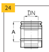
Rovný díl 0,155 m (se sponou)
