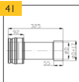
Přechod se zděří (bez spony)
