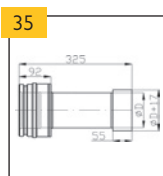
Přechod se zděří (bez spony)
