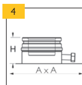
Dno s odvodem kondenzátu - do boku (se sponou)
