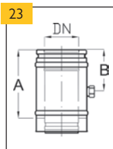
Díl s odvodem kondenzátu
