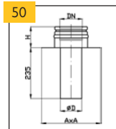
Pata nástavce
