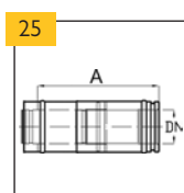
Nastav. díl kouřovodu 195 - 250 mm (se sponou)
