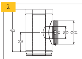
Díl s KO (bez spony)
