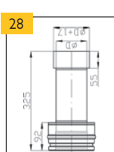
Přechod se zděří
