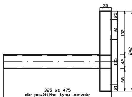
Rozměry pro založení komínu na svislou konstrukci pomocí patní konzoly Typ 570 až Typ 1504
