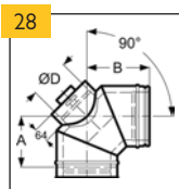
Koleno 90° s KO (se sponou)
