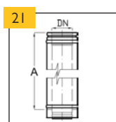
Rovný díl 0,955 m (se sponou)
