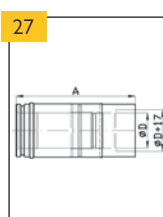
Dilatační napojovací díl
