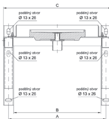
Rozměry při založení komínu na svislou konstrukci pomocí patní konzoly Typ 570 až Typ 1004
