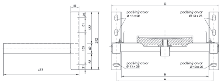
Rozměry při založení komínu na svislou konstrukci pomocí patní konzoly Typ 475
