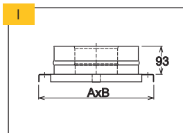
Dno s odvodem kondenzátu (bez spony)
