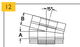
Koleno 15° (bez spony)
