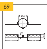
Krokový držák
