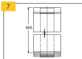
Rovný díl 955 spojený (bez spony)
