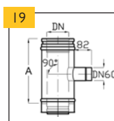
Sopouch LAS 60 (se sponou)
