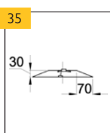
Rozeta
