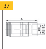
Dilatační napojovací díl
