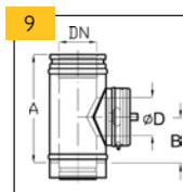
Kominový díl s KO pro přetlak (se sponou)
