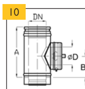
Kominový díl s KO pro podtlak (se sponou)
