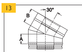
Koleno 30° (bez spony)
