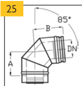
Koleno 85° (se sponou)
