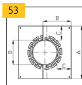
Kryt sopouchu s odvětráním 30° - 45°
