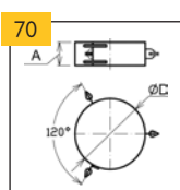
Kotvicí objímka
