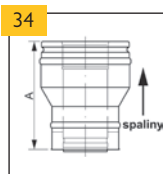
Přechodový díl ICS 25 - ICS 50 (se sponou)
