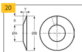
Rozeta dvouplášť
