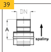
Přechodový díl ICS25 - PPL (se sponou)
