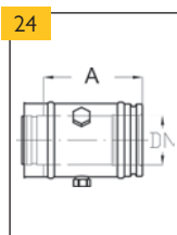
Díl pro měření
