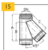
Sopouch 45° (se sponou)
