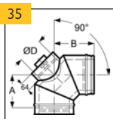
Koleno 90° s KO AQUA pro přetlak (se sponou)
