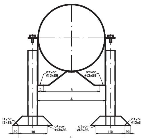
Rozměry pro založení komínu na svislou konstrukci pomocí patní konzoly Typ 570 až Typ 1504
