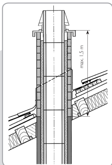
KOMÍNOVÁ HLAVA FINAL
