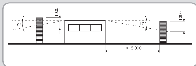
Výška komína u nástavby na ploché střeše
