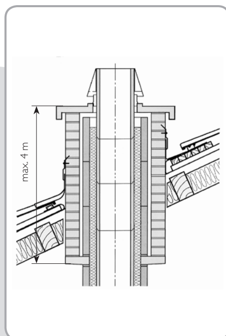
OBEZDÍVKA Z CIHEL
