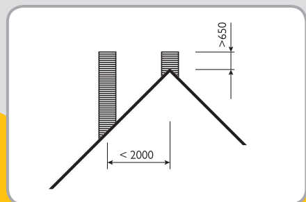
Způsob vyústění komínů nad šikmou střechou
