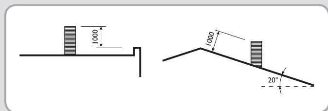
Výška komína nad plochou střechou
