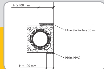
Dilatace u stěny
