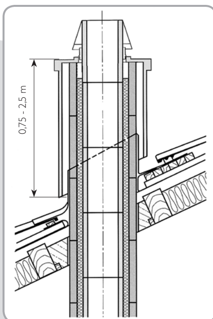
KOMÍNOVÝ PLÁŠŤ
