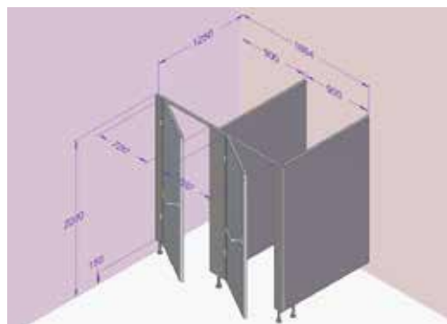
Kabina pravá, dveře levé, deska šedá obj. kód: ALU32 – E2RL-708
