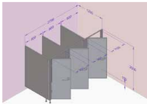
Kabina levá, dveře levé, deska šedá obj. kód: ALU32 – E3LL-708
