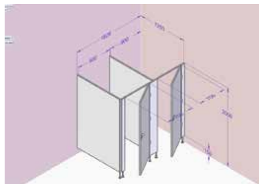
Kabina levá, dveře pravé, deska šedá obj. kód: CP13 – E2LR-708
