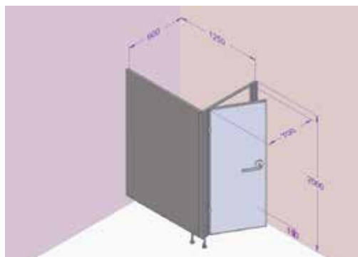
Kabina levá, dveře levé, deska šedá obj. kód: ALU32 – ELL-708
