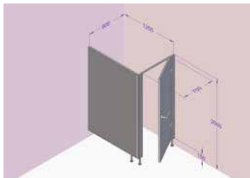
Kabina levá, dveře pravé, deska šedá obj. kód: ALU32 – ELR-708
