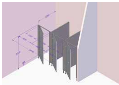
Trojkabina, dveře levé, deska šedá obj. kód: CP13 – N3L-708
