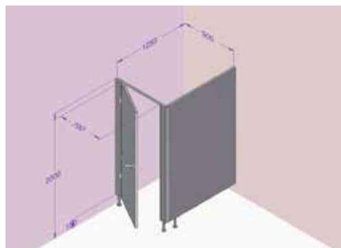
Kabina pravá, dveře levé, deska šedá obj. kód: ALU32 – ERL-708
