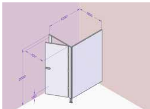
Kabina pravá, dveře pravé, deska šedá obj. kód: CP13 – ERR-708
