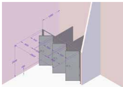
Trojkabina, dveře pravé, deska šedá obj. kód: CP13 – N3R-708
