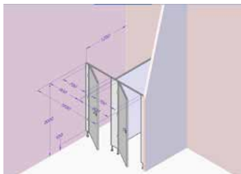
Dvojkabina, dveře levé, deska šedá obj. kód: CP13 – N2L-708
