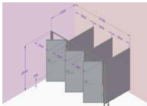
Kabina pravá, dveře pravé, deska šedá obj. kód: ALU32 – E3RR-708
