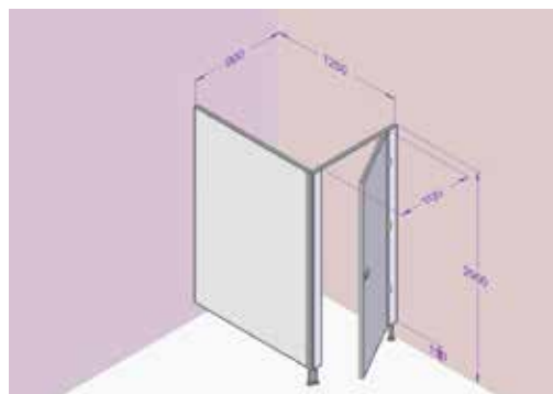
Kabina levá, dveře pravá, deska šedá obj. kód: CP13 – ELR-708
