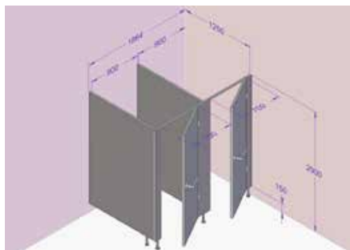
Kabina levá, dveře pravé, deska šedá obj. kód: ALU32 – E2LR-708
