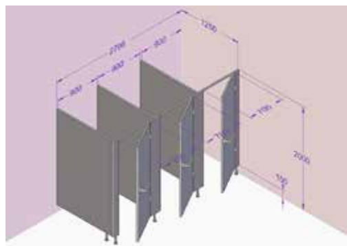
Kabina levá, dveře pravé, deska šedá obj. kód: ALU32 – E3LR-708
