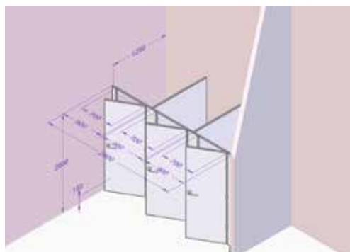
Trojkabina, dveře pravé, deska bílá obj. kód: ALU32 – N3R-980
