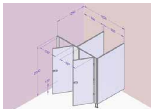
Kabina pravá, dveře pravé, deska šedá obj. kód: CP13 – E2RR-708
