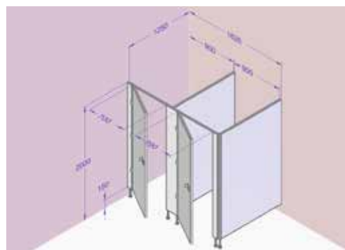
Kabina pravá, dveře levé, deska šedá obj. kód: CP13 – E2RL-708
