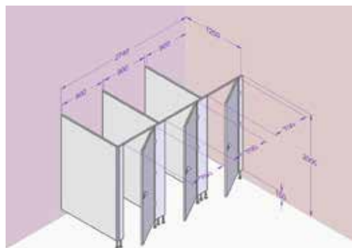
Kabina levá, dveře pravé, deska šedá obj. kód: CP13 – E3LR-708
