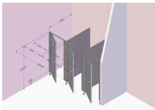
Trojkabina, dveře levé, deska šedá obj. kód: ALU32 – N3L-708
