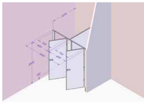
Dvojkabina, dveře pravé, deska šedá obj. kód: CP13 – N2R-708
