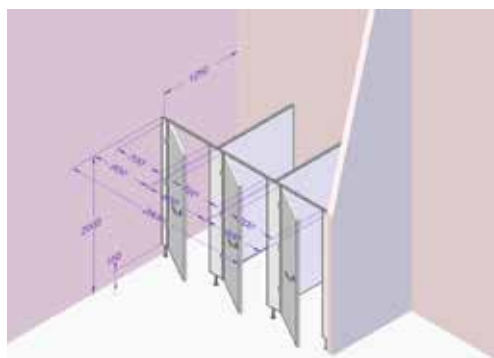
Trojkabina, dveře levé, deska bílá obj. kód: ALU32 – N3L-980
