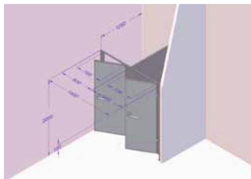
Dvojkabina, dveře pravé, deska šedá obj. kód: ALU32 – N2R-708
