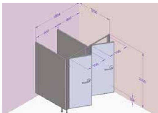
Kabina levá, dveře levé, deska šedá obj. kód: ALU32 – E2LL-708
