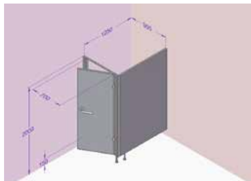
Kabina pravá, dveře pravé, deska šedá obj. kód: ALU32 – ERR-708
