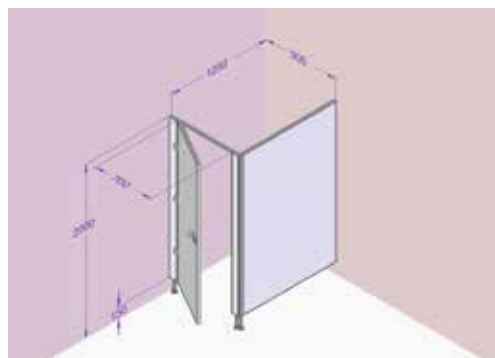
Kabina pravá, dveře levé, deska šedá obj. kód: CP13 – ERL-708
