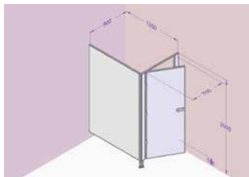
Kabina levá, dveře levé, deska šedá obj. kód: CP13 – ELL-708
