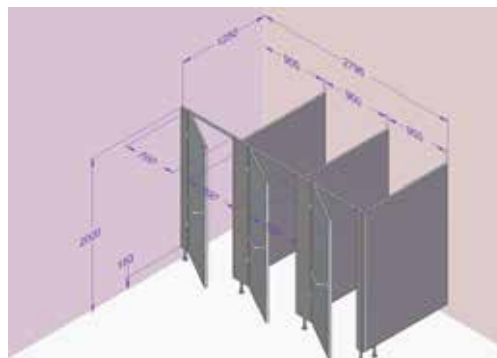
Kabina pravá, dveře levé, deska šedá obj. kód: ALU32 – E3RL-708
