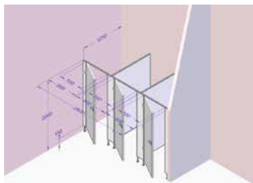
Trojkabina, dveře levé, deska bílá obj. kód: CP13 – N3L-980
