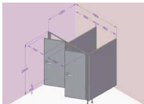
Kabina pravá, dveře pravé, deska šedá obj. kód: ALU32-E2RR-708
