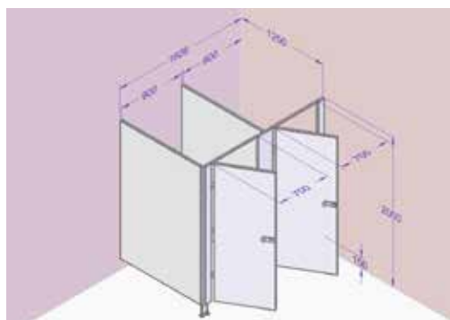
Kabina levá, dveře levé, deska šedá obj. kód: CP13 – E2LL-708
