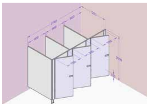
Kabina levá, dveře levé, deska šedá obj. kód: CP13 – E3LL-708
