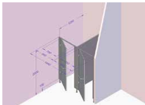
Dvojkabina, dveře levé, deska šedá obj. kód: ALU32 – N2L-708
