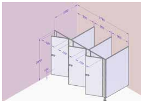
Kabina pravá, dveře pravé, deska šedá obj. kód: CP13 – E3RR-708
