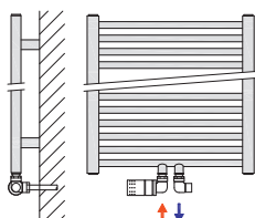
TERMOSTATICKÝ SET ÚHLOVÝ - TRIAXIÁLNÍ
