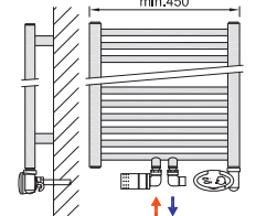
FORTE + TERMOSTATICKÝ SET ÚHLOVÝ - TRIAXIÁLNÍ
