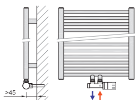
ROHOVÝ STŘEDOVÝ TERMOSTATICKÝ VENTIL
