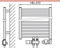
FORTE + PŘÍMÝ STŘEDOVÝ TERMOSTATICKÝ VENTIL
