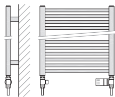
TERMOSTATICKÝ SET PŘÍMÝ
