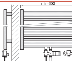
FORTE + PŘÍMÝ STŘEDOVÝ TERMOSTATICKÝ VENTIL
